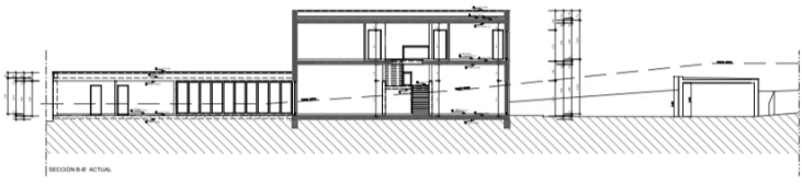
SECCION B-B ACTUAL
