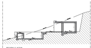
SECCION C-C ACTUAL
